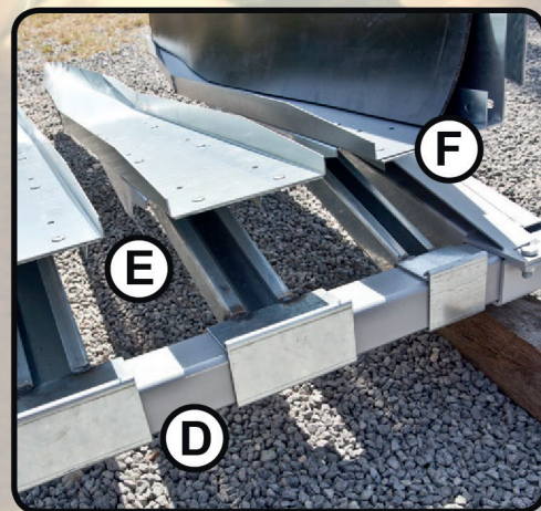
Le tube carré D soutient les plateaux E . Une bande caoutchoutée F vient faire la jonction entre les plateaux de rive et les diviseurs.
