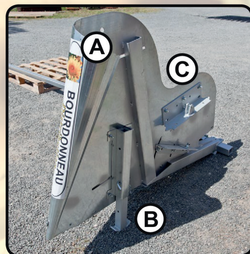
Le diviseur A , sa béquille B et l'attache du tendeur à cliquer C
